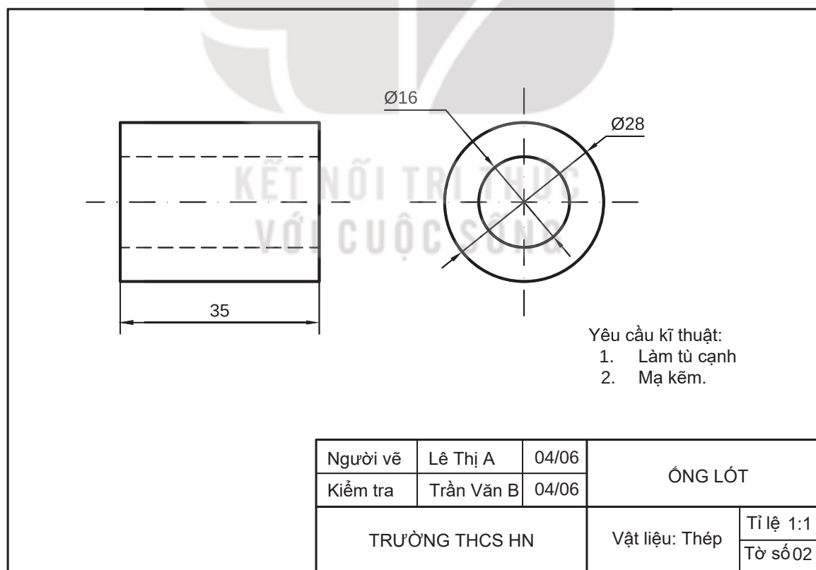
Hình 3.5. Bản vẽ ống lót
