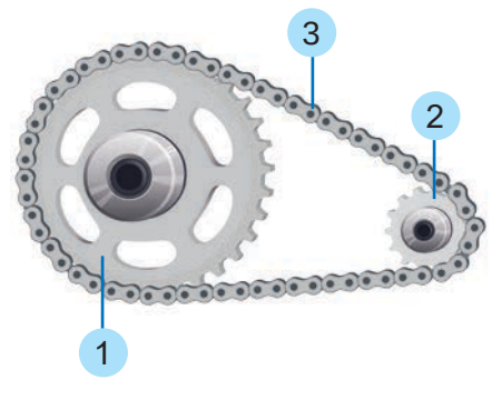
b) Truyền động xích
