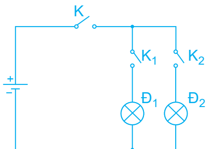
Hình 14.1. Mạch điện đơn giản
