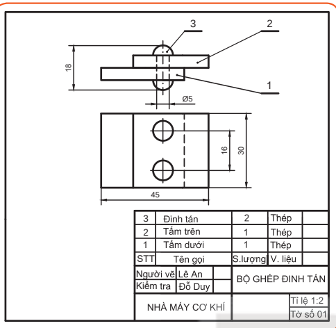
Hình 4.1. Bản vẽ lắp bộ ghép đinh tán
