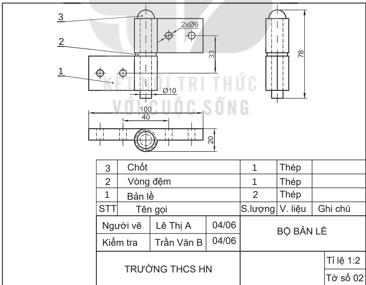
Hình 4.6. Bản vẽ lắp của bộ bản lề
