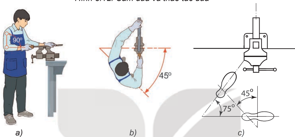
Hình 8.13. Tư thế dũa và vị trí chân
