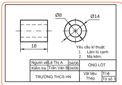
Hình 3.1. Bản vẽ chi tiết
