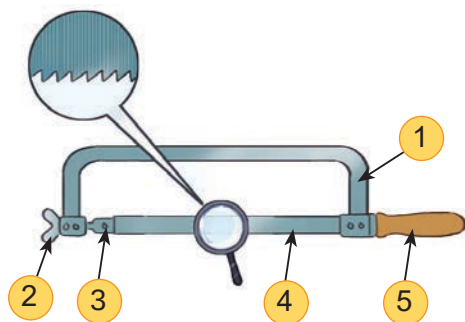
a) Cấu tạo cưa tay
