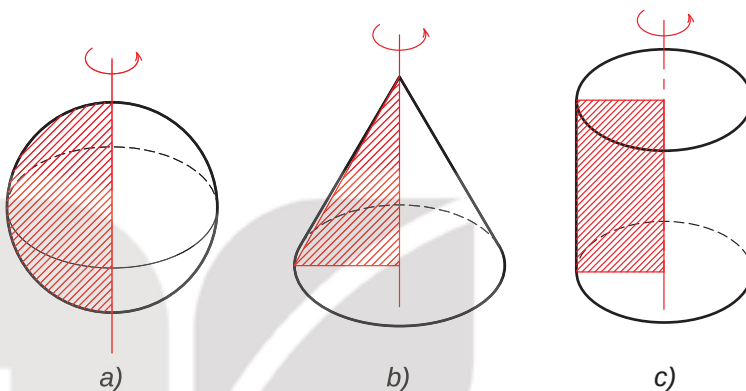
Hình 2.12. Các khối tròn xoay thường gặp
