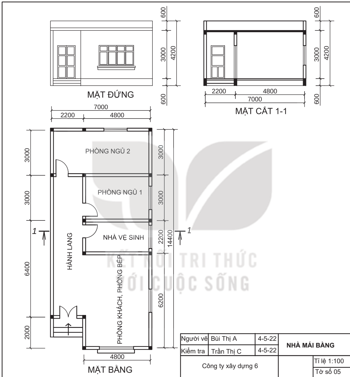
Hình 5.4. Bản vẽ ngôi nhà mái bằng
