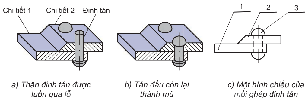
Hình 4.3. Mối ghép đinh tán
