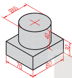
Hình 2.19. Gối đỡ
