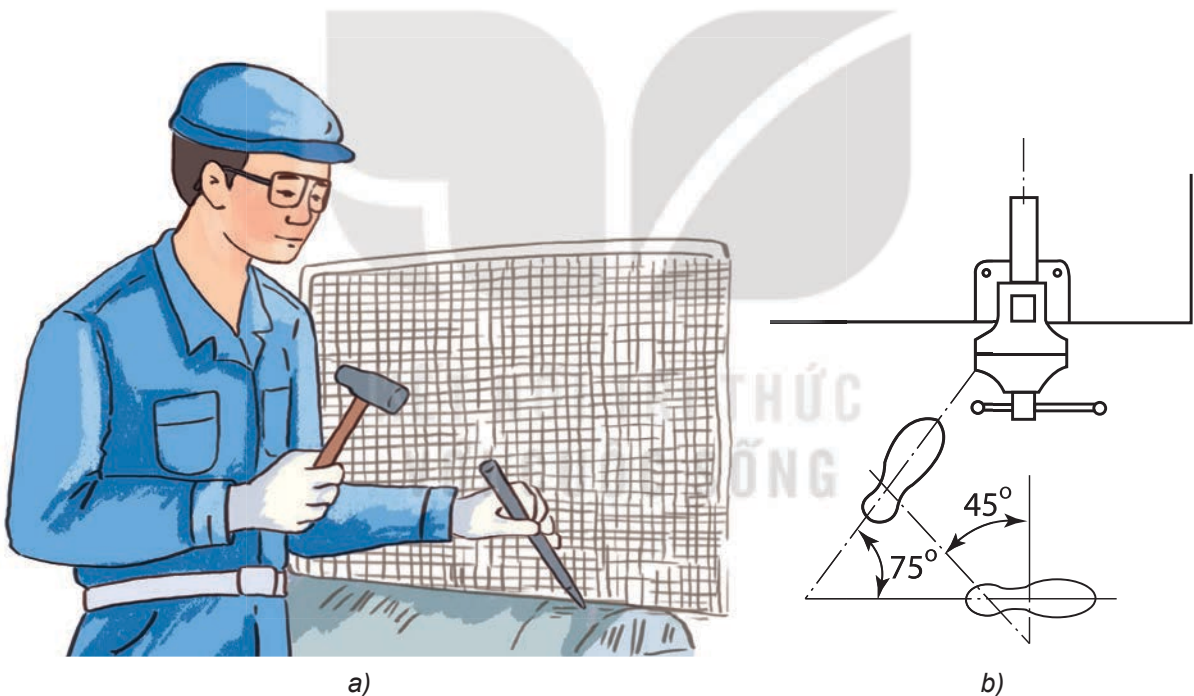
Hình 8.10. Tư thế đục và vị trí chân
