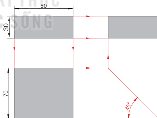
Hình 2.22. Vẽ khối hộp chữ nhật (1)
