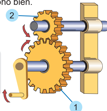
a) Truyền động bánh răng
