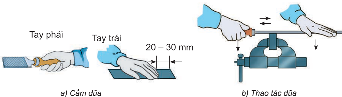
Hình 8.12. Cầm dũa và thao tác dũa
