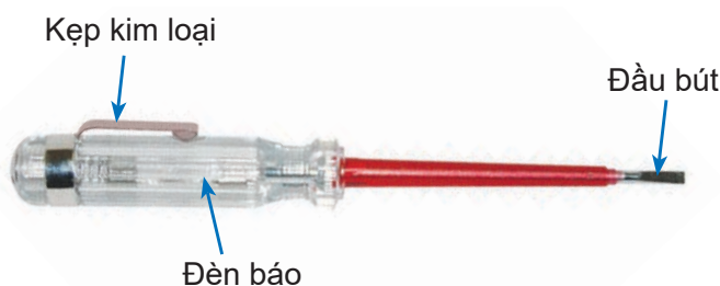
Hình 12.6. Cấu tạo của bút thử điện
