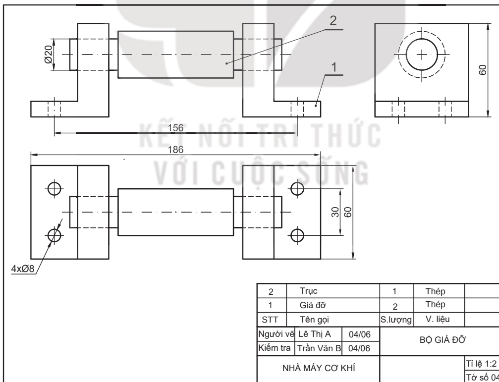
Hình 4.8. Bản vẽ lắp bộ giá đỡ
