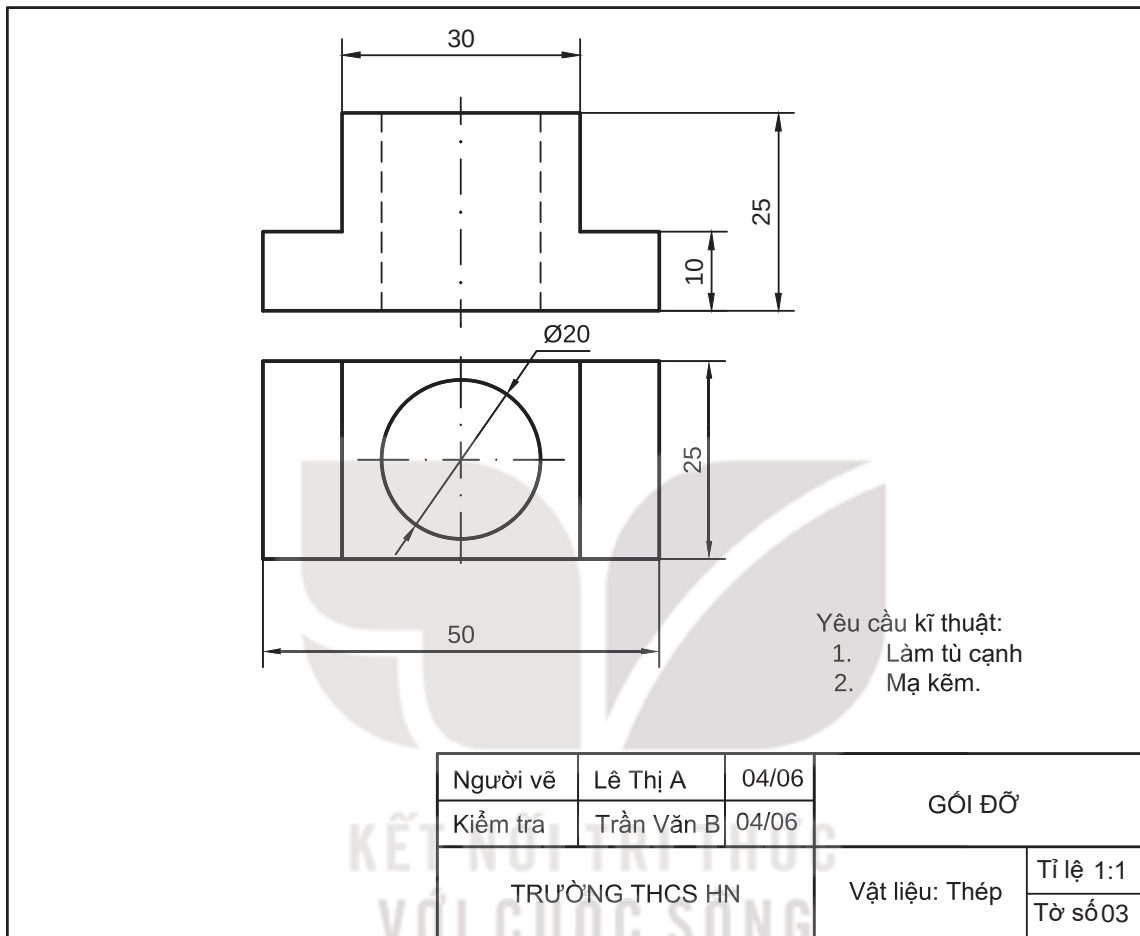
Hình 3.6. Bản vẽ gối đỡ
